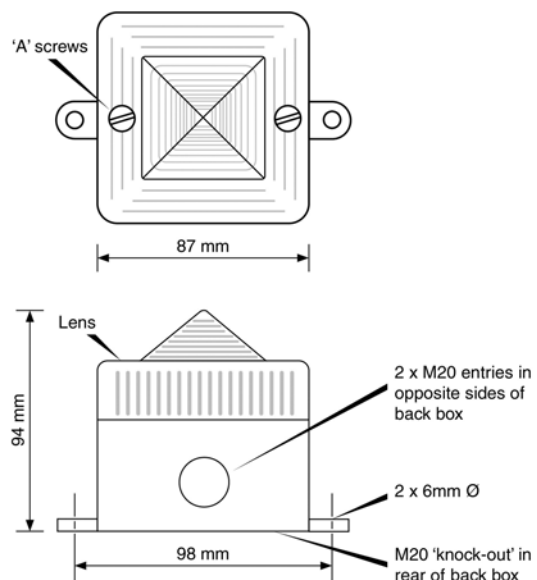
Fig 2 BA386 dimensions
