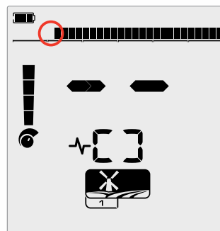
ID de objetivo rechazados 1 a 4 en el patrón de discriminación para perfiles de búsqueda en Modo Campo.
