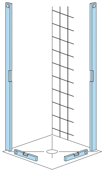
Bodenebene Montage
