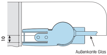
Außenkante Glas
