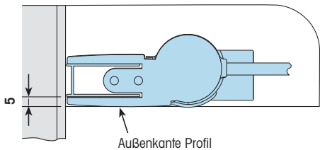
Außenkante Profil
