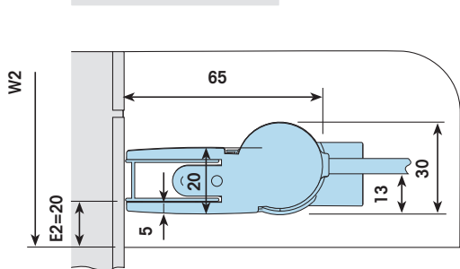
Montage auf Duschwanne
