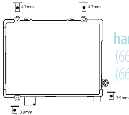
thermal module clamp (boomerang, 922-8316)
