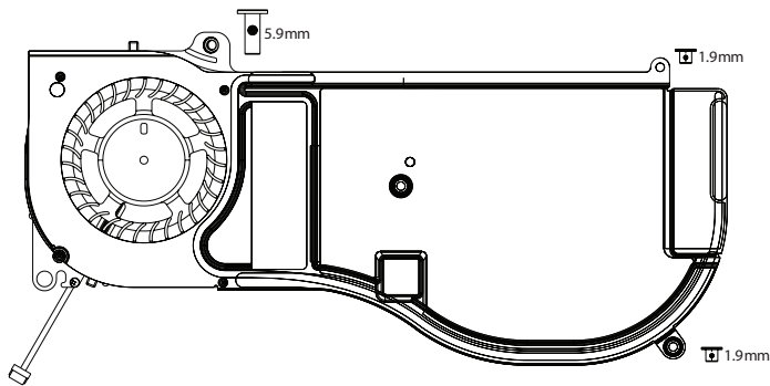
thermal module assy (922-8316)
