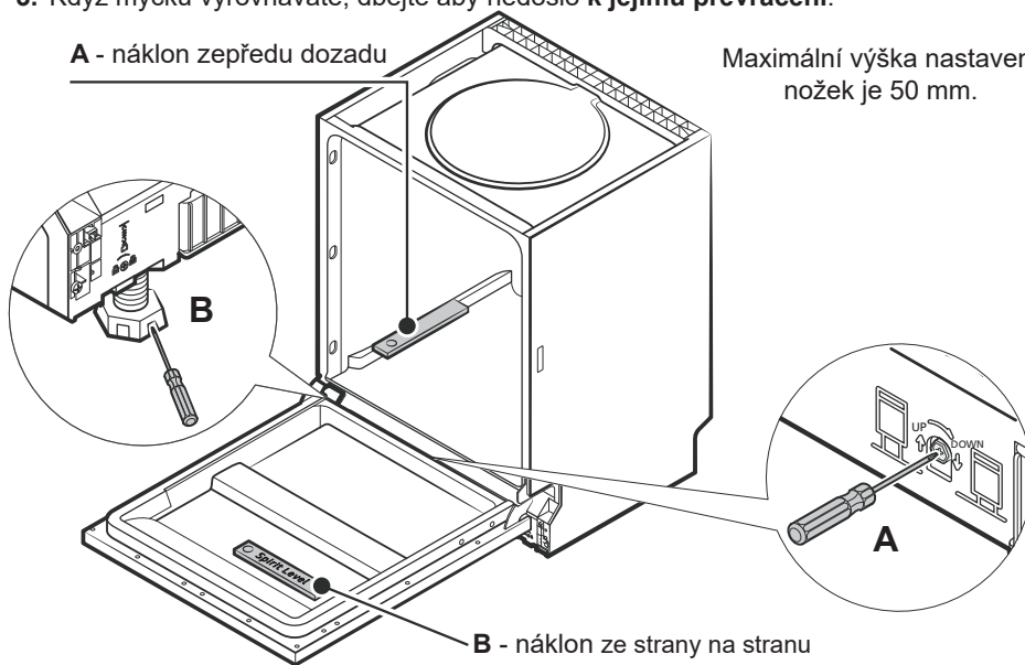
Obrázek 6 - vyrovnání myčky
