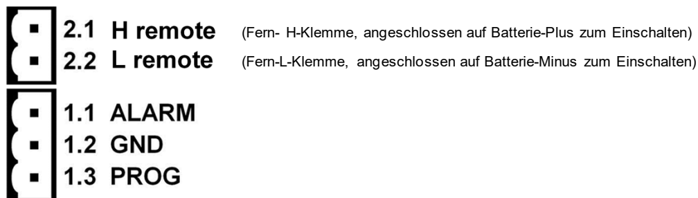
Abbildung 3: Steckverbinder und Pin-Nummerierung
