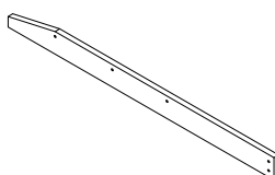
Right Under Trundle Connect Bar 1 pc Barre de connexion juste sous le lit gigogne 1pièce
