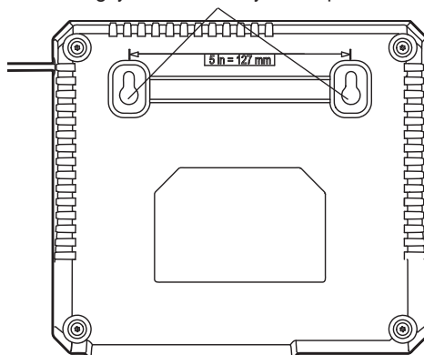
Fig. 3 Agujeros de montaje en la pared
