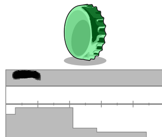
Capsule B sur la tranche (à la verticale). Dans ce cas, le détecteur ne voit que très peu la forme plate de l'objet et la réponse se situe dans la région ferreuse supérieure.
