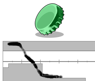
Capsule B inclinée à 45 degrés. Dans ce cas, le détecteur voit à la fois la forme plate de l'objet et ses côtés plus étroits, qui ont tendance à apparaître dans la région ferreuse supérieure.
