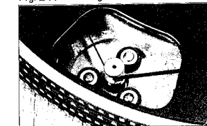
Fig. 2-A Looping the Belt Abb. 2-A Treibriemeneneinsatz Fig. 2-A Bouclage de la Courroie
