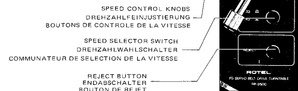
Fig. 8 Control Panel Abb. 8 Bedienungsfeld Fig. 8 Paneau de Contrôle
