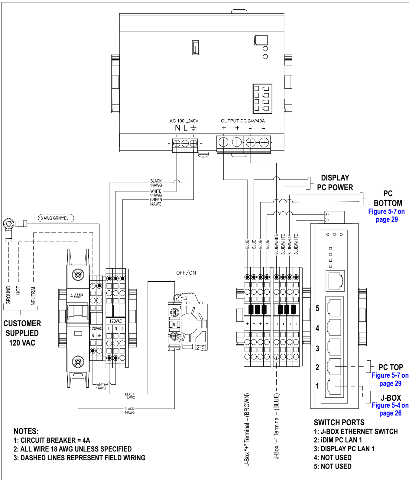
Figure 5-6. Kiosk Wiring
