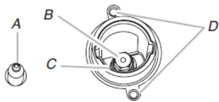
A. Electrodo encendedor B. Tornillo del orificio C. Soporte del tornillo de los orificios D. Tornillos
