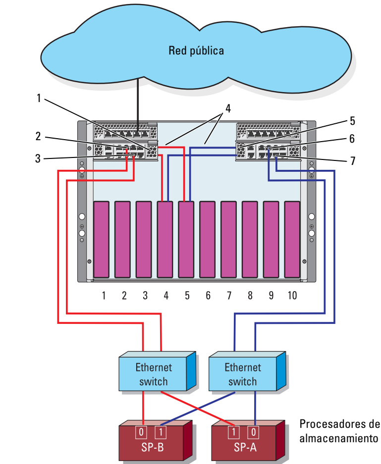
Ilustración 2-10. Clúster de conexión mediante red iSCSI externo con módulos de paso a través Ethernet incorporados
