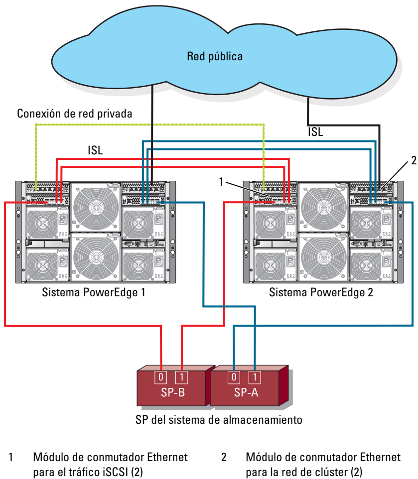
Ilustración 2-8. Configuración del clúster con dos alojamientos del servidor PowerEdge y un sistema de almacenamiento
