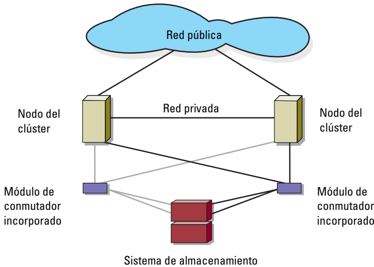
Ilustración 1-4. Clúster de conexión mediante conmutador conectado a una SAN externa mediante módulos de conmutador incorporados
