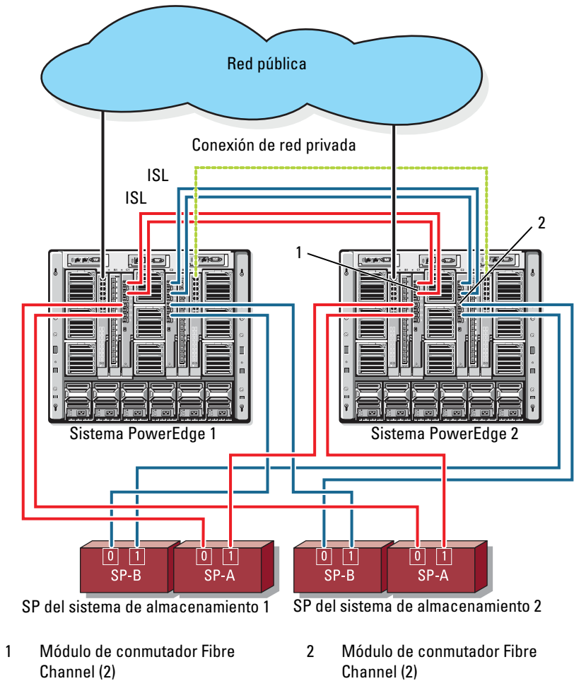
Ilustración 2-9. Dos alojamientos del servidor PowerEdge conectados a dos sistemas de almacenamiento
