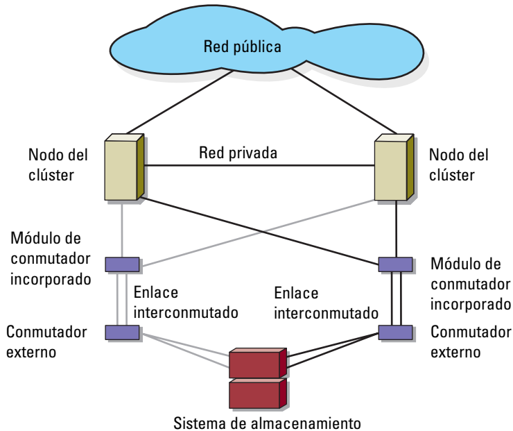
Ilustración 1-6. Clúster de conexión mediante conmutador conectado a una SAN externa mediante módulos de conmutador incorporados
