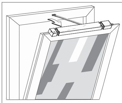
Abb. 1: KCDL Flügelmontage am Kipp- oder Drehfenster
