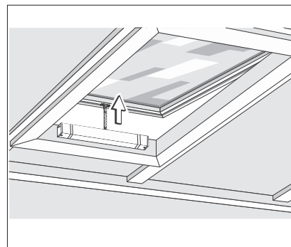
Abb. 3: KCDL Rahmenmontage am Dachfenster
