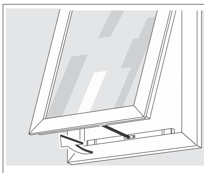
Abb. 2: KCDL Rahmenmontage am Klappfenster
