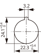
开孔尺寸
