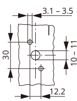
开孔尺寸
