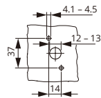
门开孔尺寸
