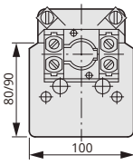
开孔尺寸（底座）
