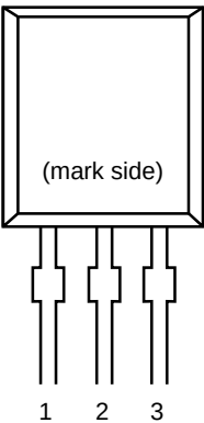
• TO-92
