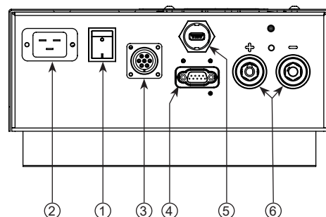
GYSFLASH 148.12 CNT
