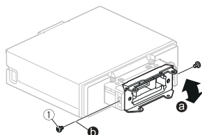
① Tornillo de cabeza fijadora (4 mm × 6 mm)
