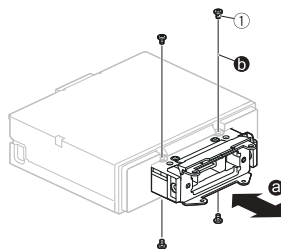
① Tornillo de cabeza fijadora (4 mm × 6 mm)
