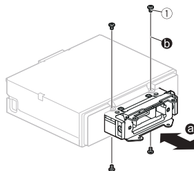
① Vis de fixation (4 mm × 6 mm)
