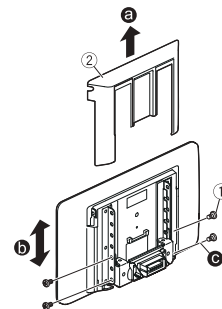
① Klemmkopfschraube (4 mm × 6 mm) ② Monitorabdeckung
