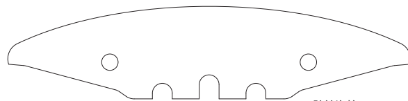
防撞泡棉 ×1 Bumper 130005
