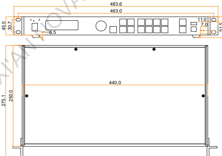
VX4 's dimension (Unit:mm)
