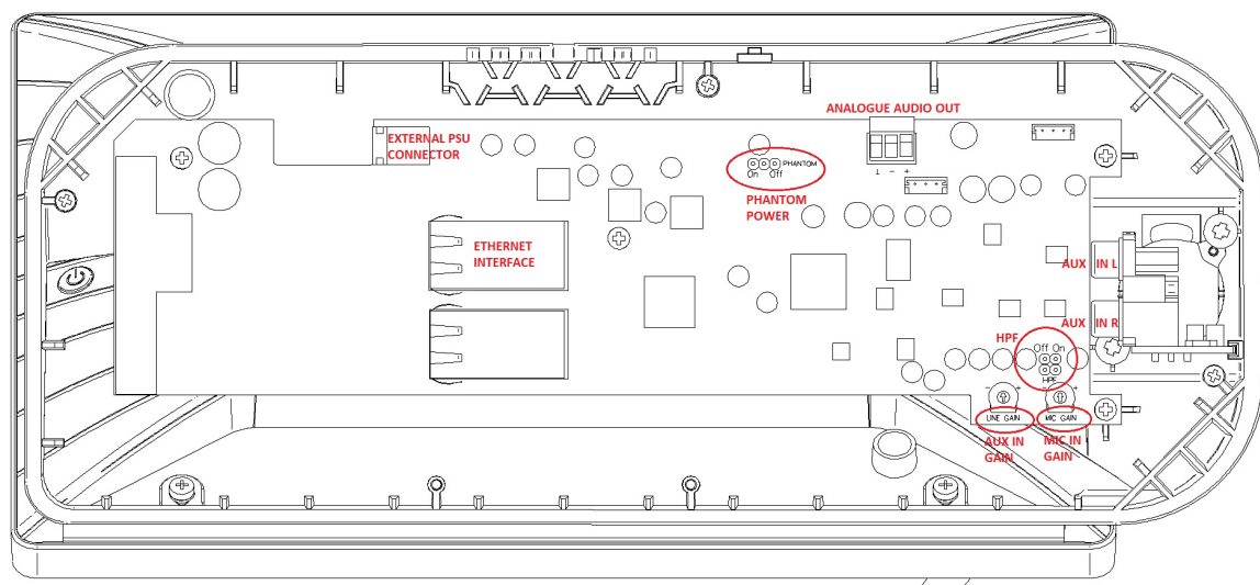
Vue intérieure du PAGENET, après retrait de la plaque métallique inférieure
