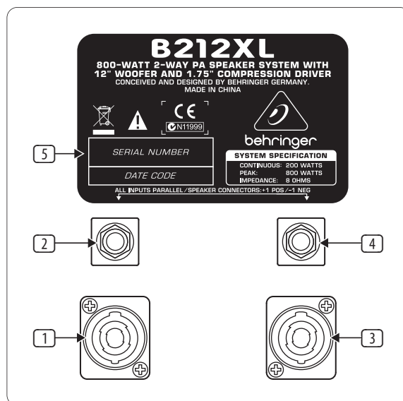
Kuva 2.1: Liitännät (B212XL ja B215XL)
