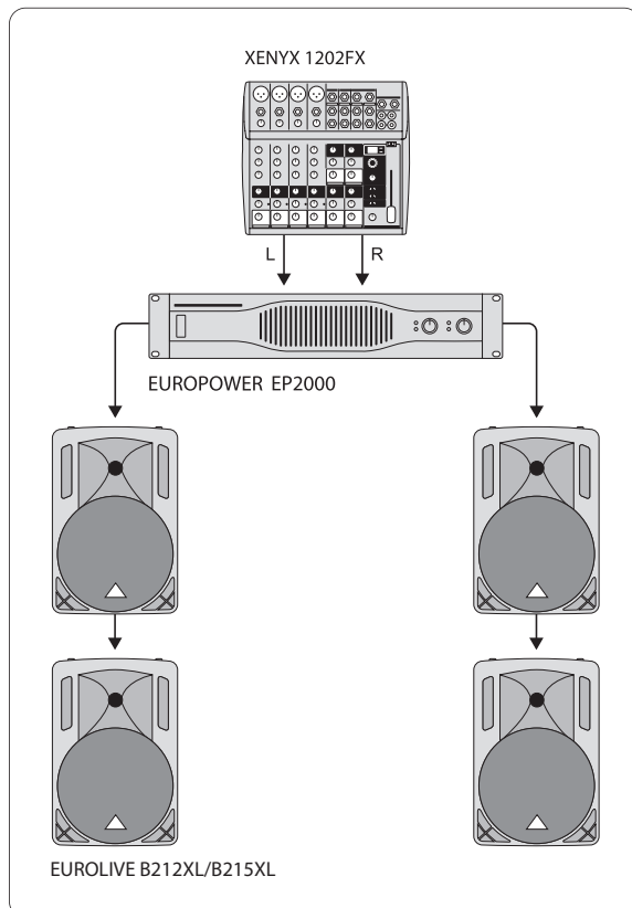
Kuva 5.2: Useampien B212XL/B215XL-kaiuttimien johdotus
