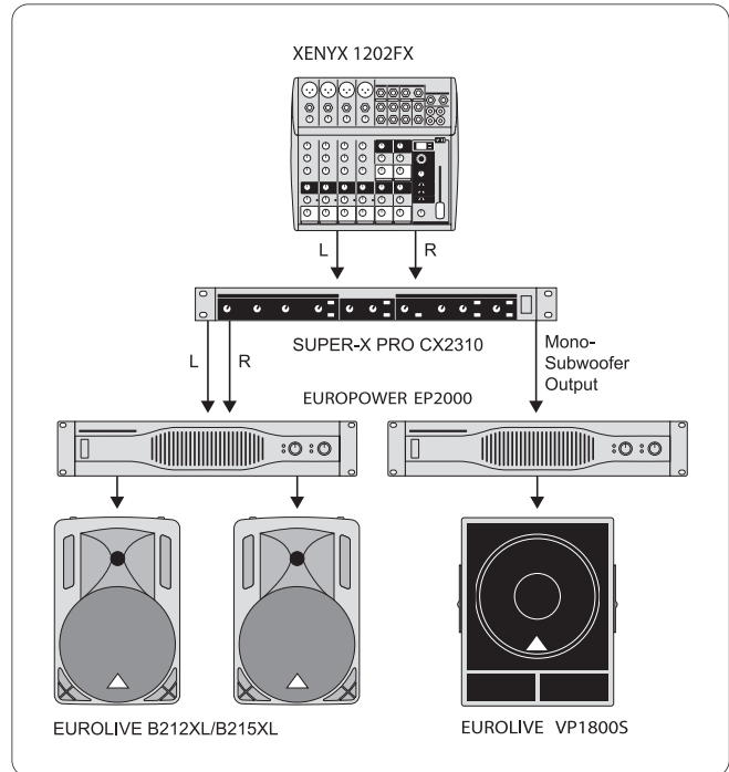
Kuva 5.3: Stereokäyttö subwooferin kera
