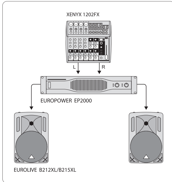
Kuva 5.1: Full Range-stereokäyttö
