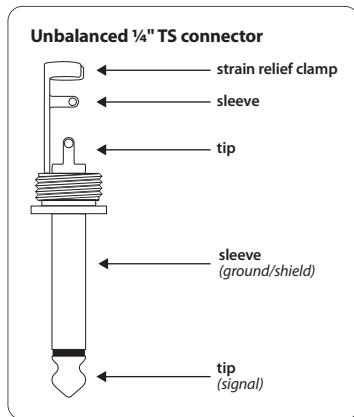
Kuva 6.2: 6,3-mm-mono-jakkipistoke
