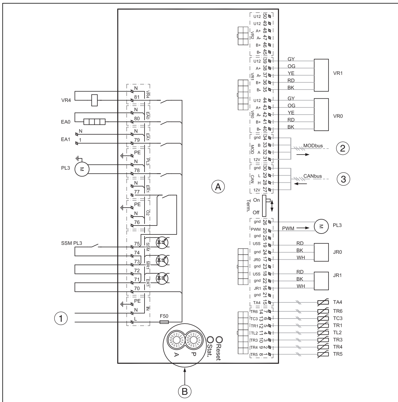
Fig. 26 Wiring diagram I/O module
