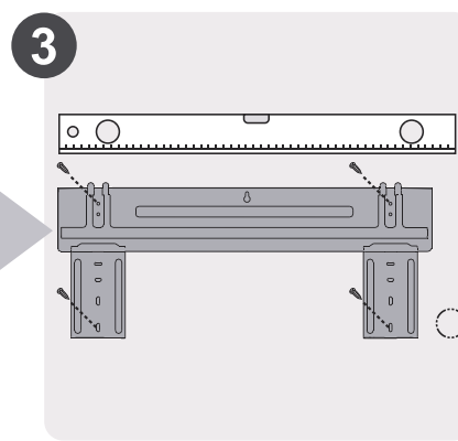
Συνδέστε την πλάκα συναρμολόγησης
