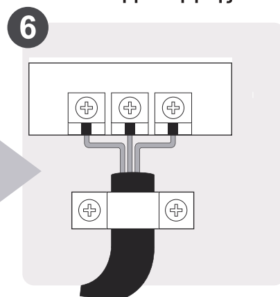
Συνδέστε την καλωδίωση (δεν ισχύει για ορισμένες τοποθεσίες στη Βόρεια Αμερική)
