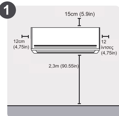
Επιλέξτε Τοποθεσία εγκατάστασης
