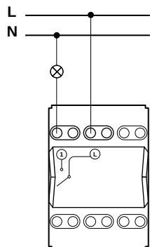
Выключатель
