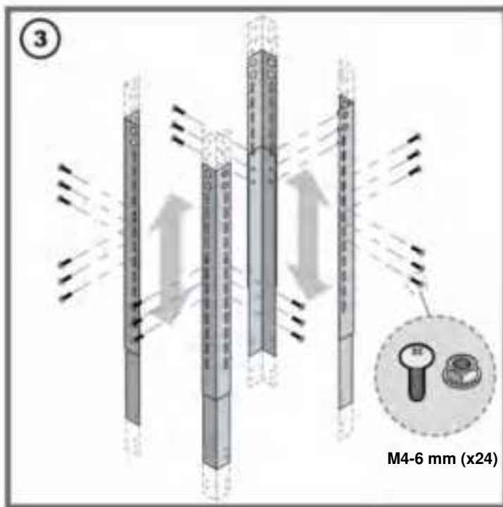
(3) Bestäm den höjd som krävs för att stödja förlängningarna. Fäst varje stöddarm med skruvar med låsmuttrar, 3 skruvar per sida rekommenderas, inte mindre än 2 skruvar per sida om höjjustering krävs.
