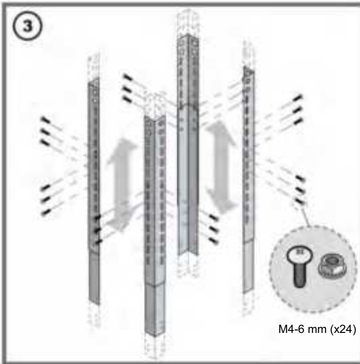
(3) Determine la altura necesaria para soportar las extensiones. Asegure cada brazo de soporte con tornillos con contratuercas, se recomiendan 3 tornillos por lado, no menos de 2 tornillos por lado si se requiere ajuste de altura.
