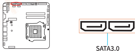
图2-7 SATA接口
