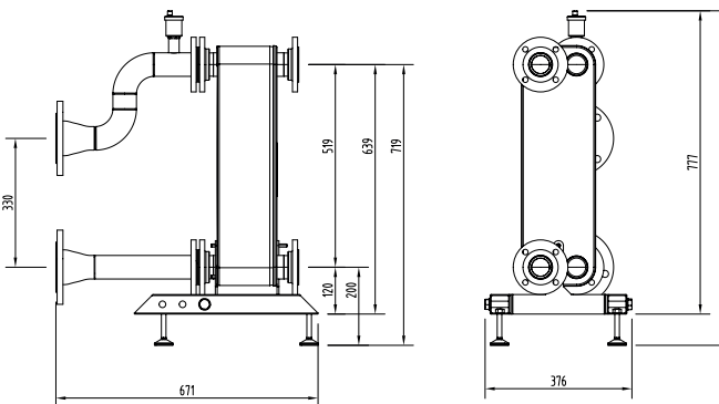
222225 DN80
