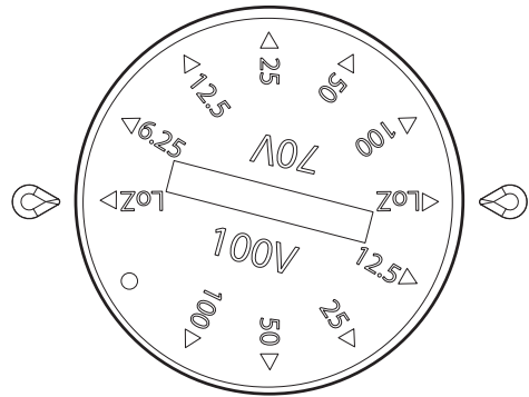
Afb.1 VLS 5 moduskeuzeschakelaar
