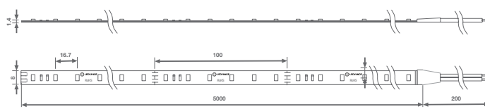
Dimension: LM SV 200 RGB DC P 36W
