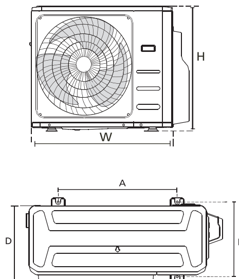
Types et Spécifications de l'Unité Extérieure
