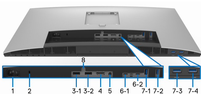
底视图（无显示器支架）
