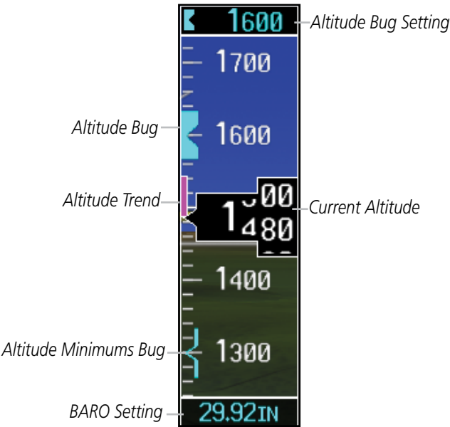
Altitude Tape
