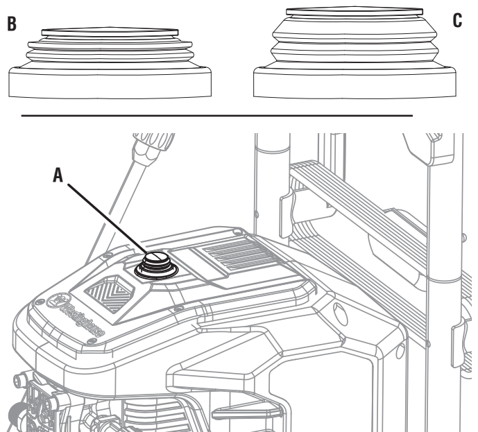
A - Interruptor encendido / apagado B - Posición encendido C - Posición apagado
