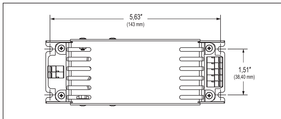
Figura 2. Dimensiones del adaptador LED Smart Sync
