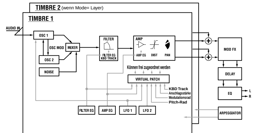
BLOCKSCHALTBILD DER SYNTHI-PROGRAMMS
