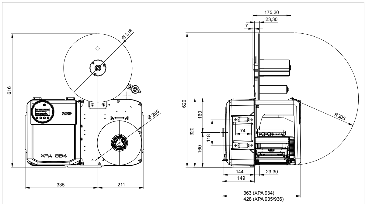
Bild 4: Abmessungen der XPA 934 LH mit Compact-Abwickler.
