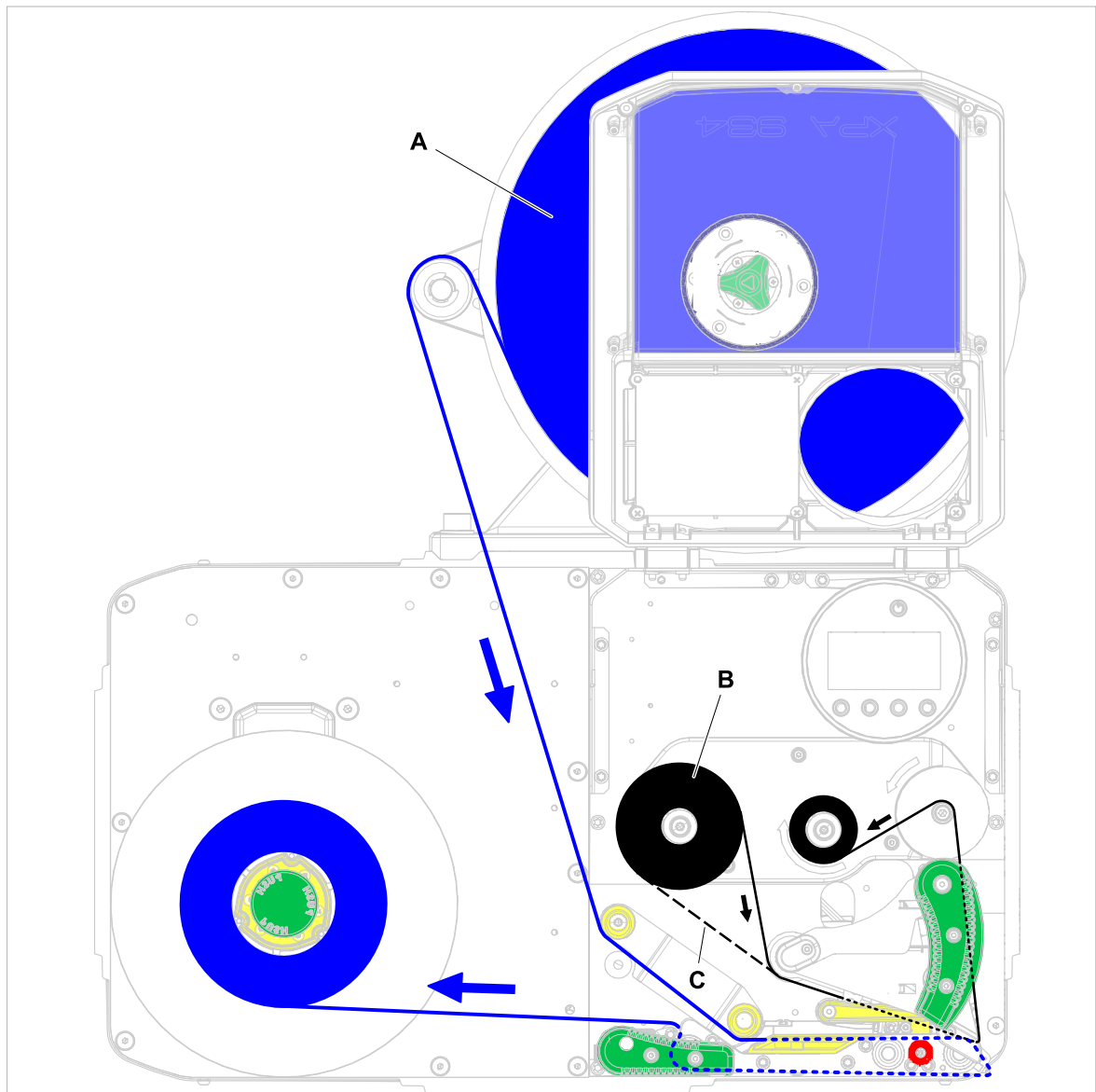
Bild 46: Fädelschema für Etikettenmaterial (A) und Thermotransfer-Folie (B) am XPA 93x RH mit Abwickler „Pro 300“ mit nach rechts gerichtetem Arm. Nach innen gewickeltes Etikettenmaterial kann mit dieser Konfiguration nicht verwendet werden. C = Pfad für mit der Farbseite nach außen gewickelte Folie.
