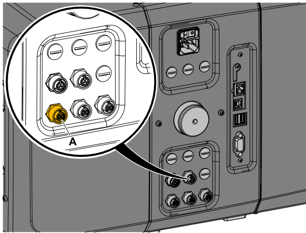
Bild 34: Anschluss (A) für den Startsensor an der BasicIO-Platine.
