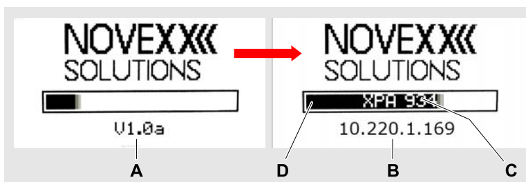
Bild 36: Wechselnde Informationen auf der Anzeige während des Hochfahrens: A Firmware-Version, B (Optional) IP-Adresse (falls Ethernet als Datenschnittstelle gewählt ist), C Druckertyp, D Fortschrittsbalken.
