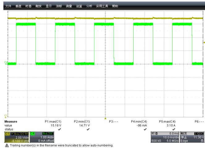
Figure 35: 264Vac / 60Hz 15V/ 0~3A \Delta V=47mV
