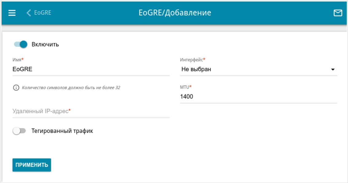
Рисунок 116. Страница добавления EoGRE-туннеля.
