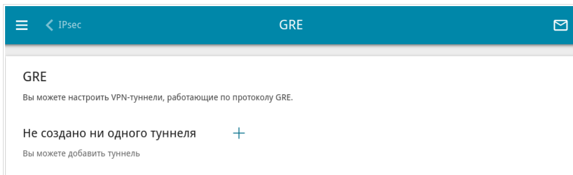
Рисунок 107. Страница VPN / GRE .
