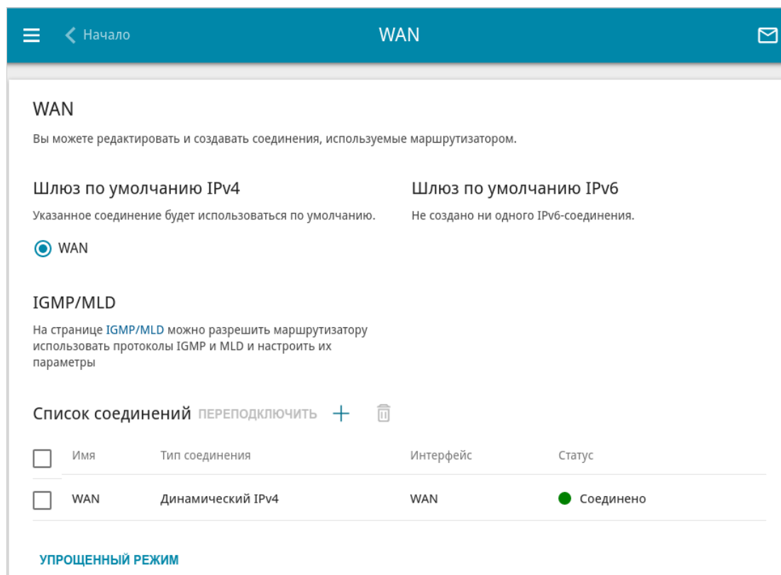
Рисунок 65. Страница Настройка соединений / WAN . Расширенный режим.
