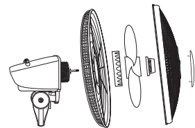
1. Ensamble la cabeza del ventilador
