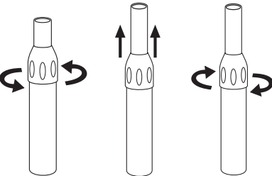
2. Afloje la tuerca, extienda la tubería hacia arriba, apriete la tuerca
