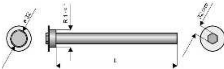
Anode isolée en magnésium - connexion taille et longueur
