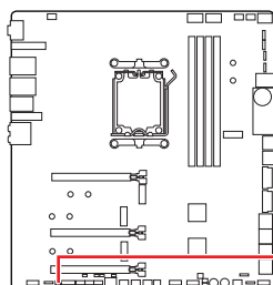
JPWRLED1 - LED電源入力
