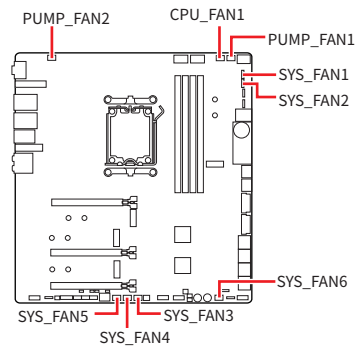
PWM 模式接腳定義
