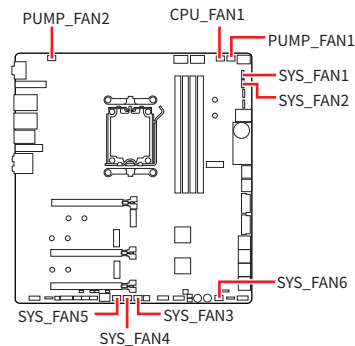
PWM 模式针脚定义
