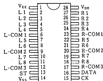
NJU7313AL
