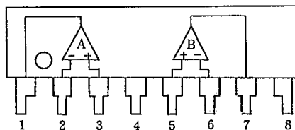
NJM5532L
