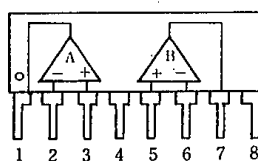
NJM2068L
