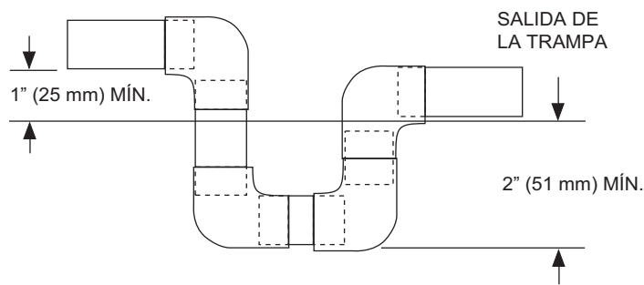
Fig. 9 – Trampa de condensado de PVC
