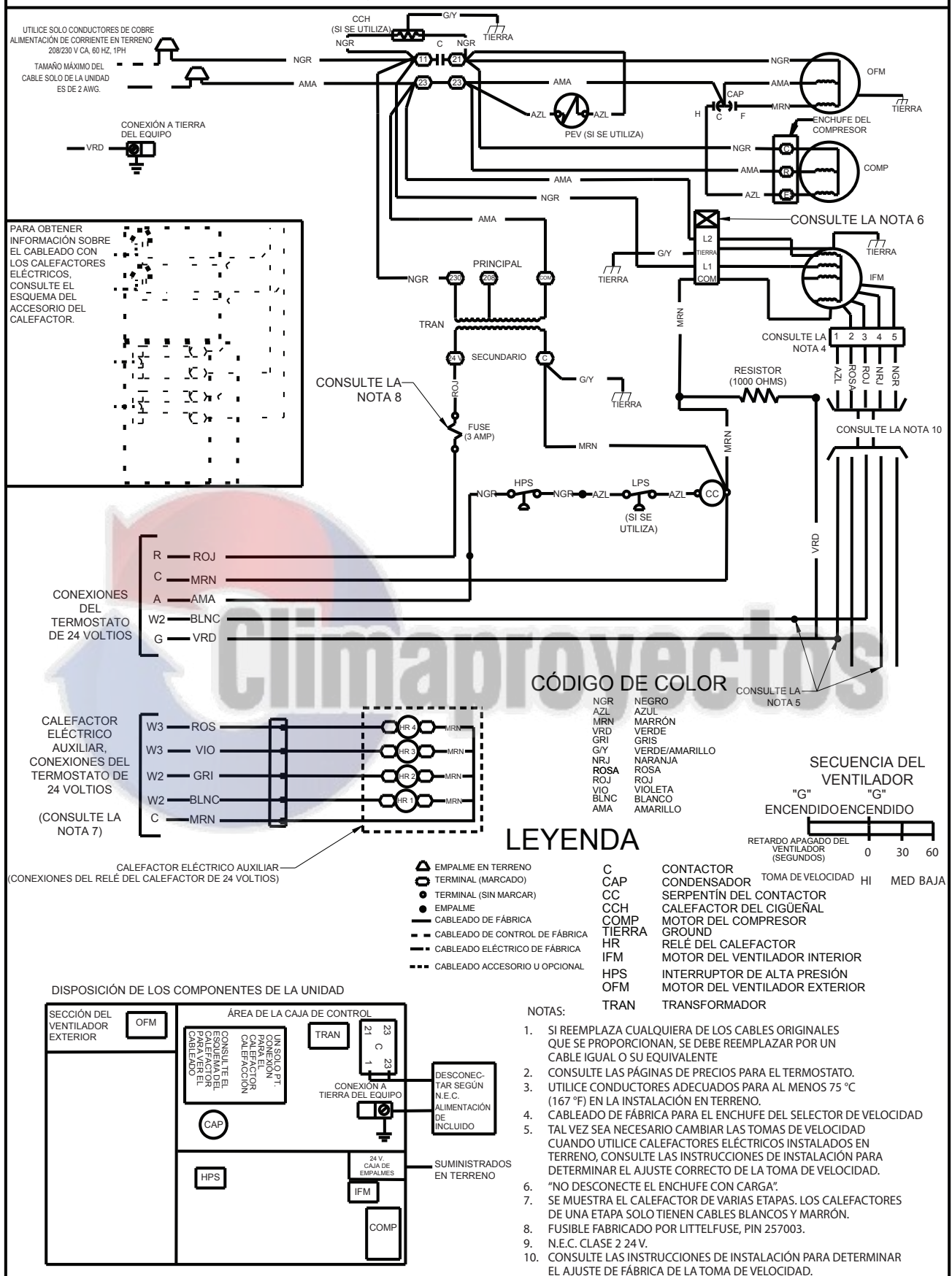
Fig. 14 – Esquema eléctrico de conexión monofásico
