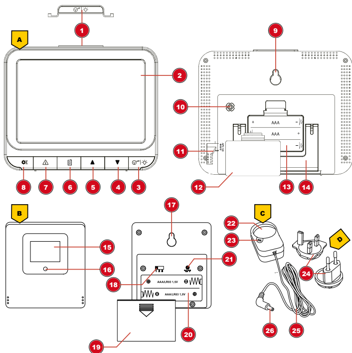
Figura 1: Tutte le parti della stazione base (in alto), del sensore radio (in basso a sinistra) e dell'alimentatore inclusi gli adattatori di spina (in basso a destra)
