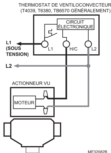
Fig. 11. Câblage typique de l'actionneur série VU40.
