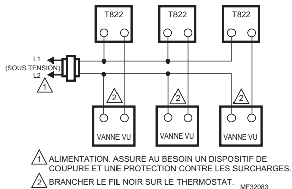
Fig. 12. Thermostat T822, raccordement de l'actionneur série VU80.
