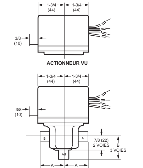
DIMENSIONS DE VANNE VU53 ET VU54 AVEC ACTIONNEUR
