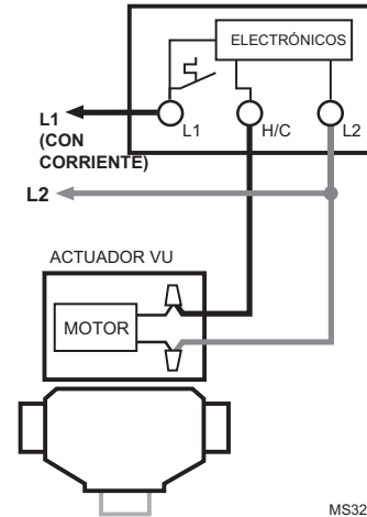
Fig. 12. Cableado típico para el actuador de la serie VU40.
