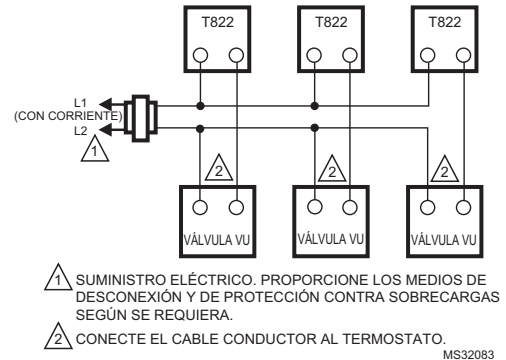
Fig. 13. Conexiones del actuador serie VU80 y del termostato serie T822.
