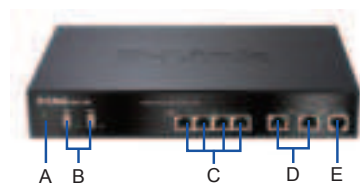
Figura 1. Pannello frontale del dispositivo DWC-1000
