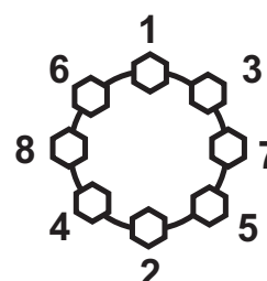
8-Lug Nuts
