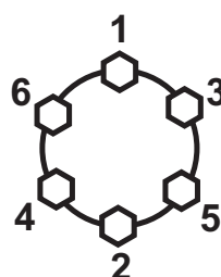
6-Lug Nuts
