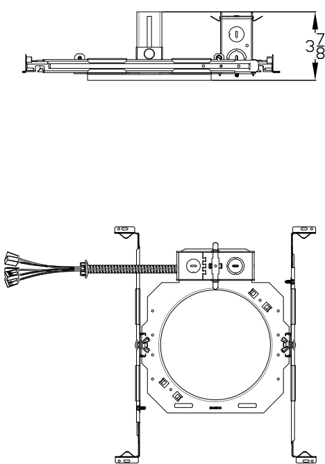
4" New Construction Frame, 18" conduit
