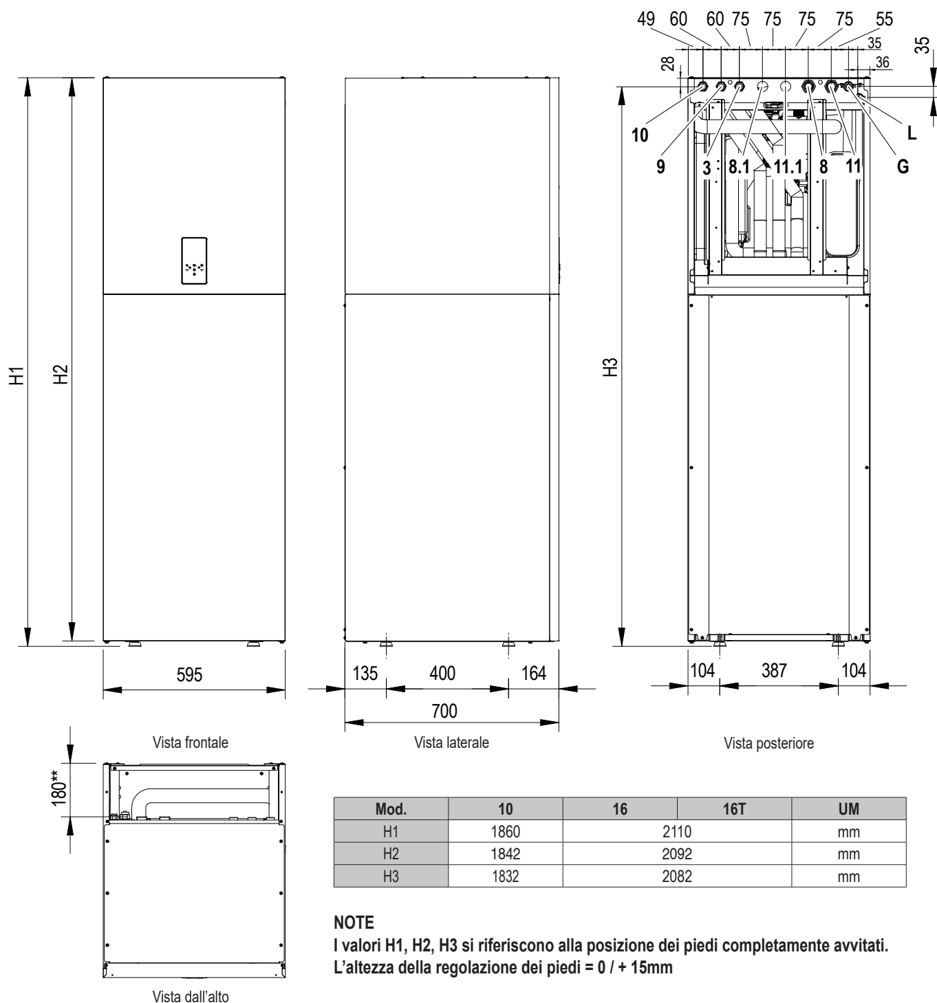
fig. 3 - dati dimensionali e connessioni
