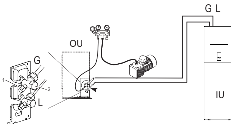
fig. 14 - Spurgo aria con pompa del vuoto
